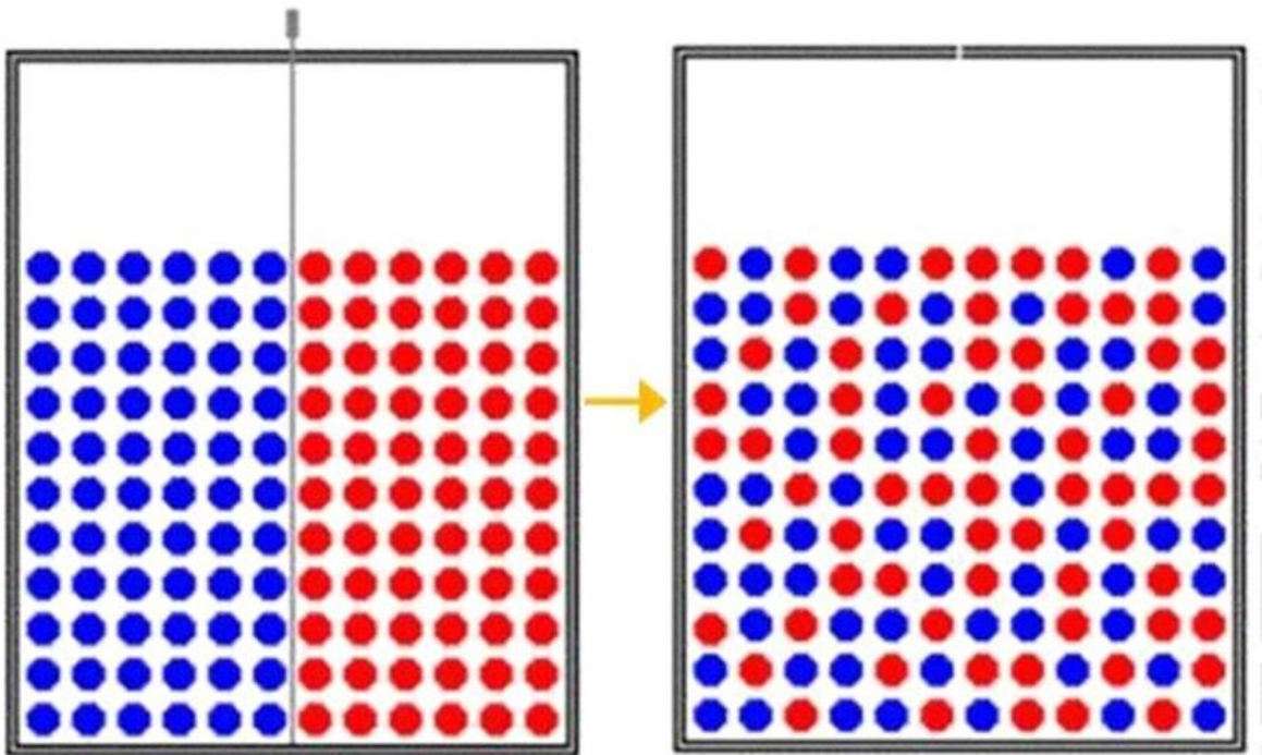
熵增定律/热力学第二定律 东方号
